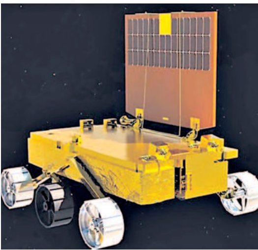
ప్రజ్ఞాన్ రోవర్
