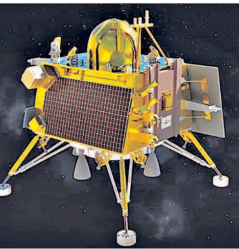
విక్రమ్ ల్యాండ్
